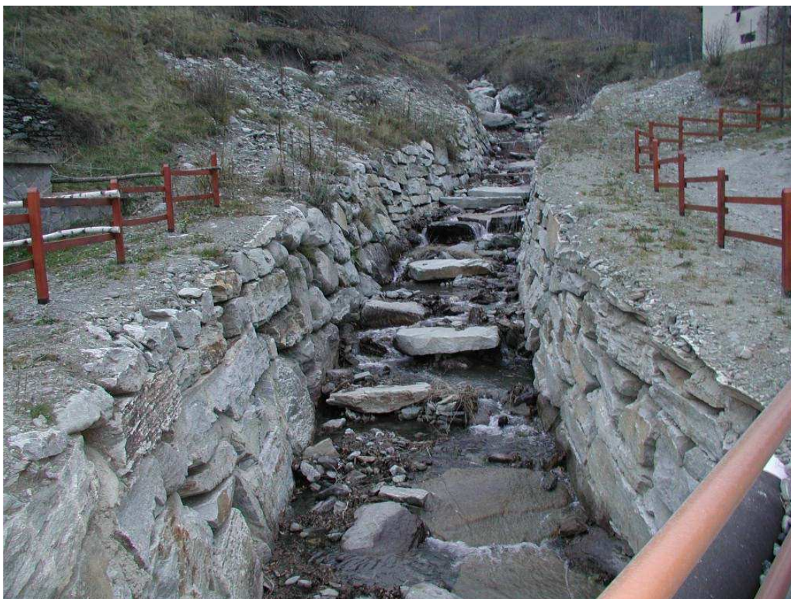
Foto 008 – Opere BELTDS008 e BATTDS009 . Da valle, in corrispondenza dell'attraversamento BELTAG002 sul Rio di Cristove.
