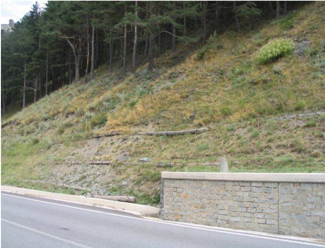
Foto 001 – Opera PENNOSS001 . Ripresa da valle lungo la SR 23 tra Depot e Fenestrelle.
