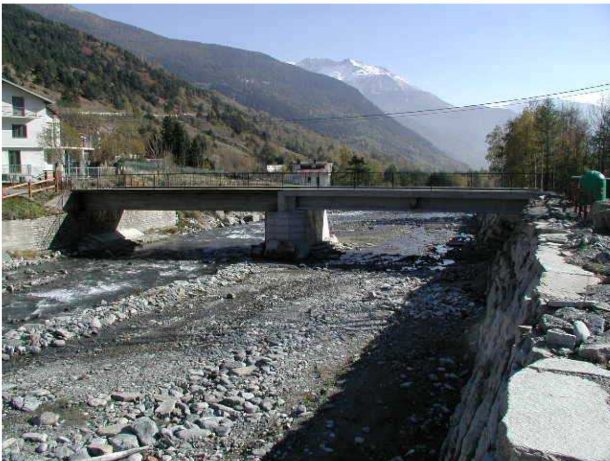
Foto 012 – Opera BELTPO012 . Da valle sponda sinistra del T. Chisone, lavori di ampliamento ultimati.
