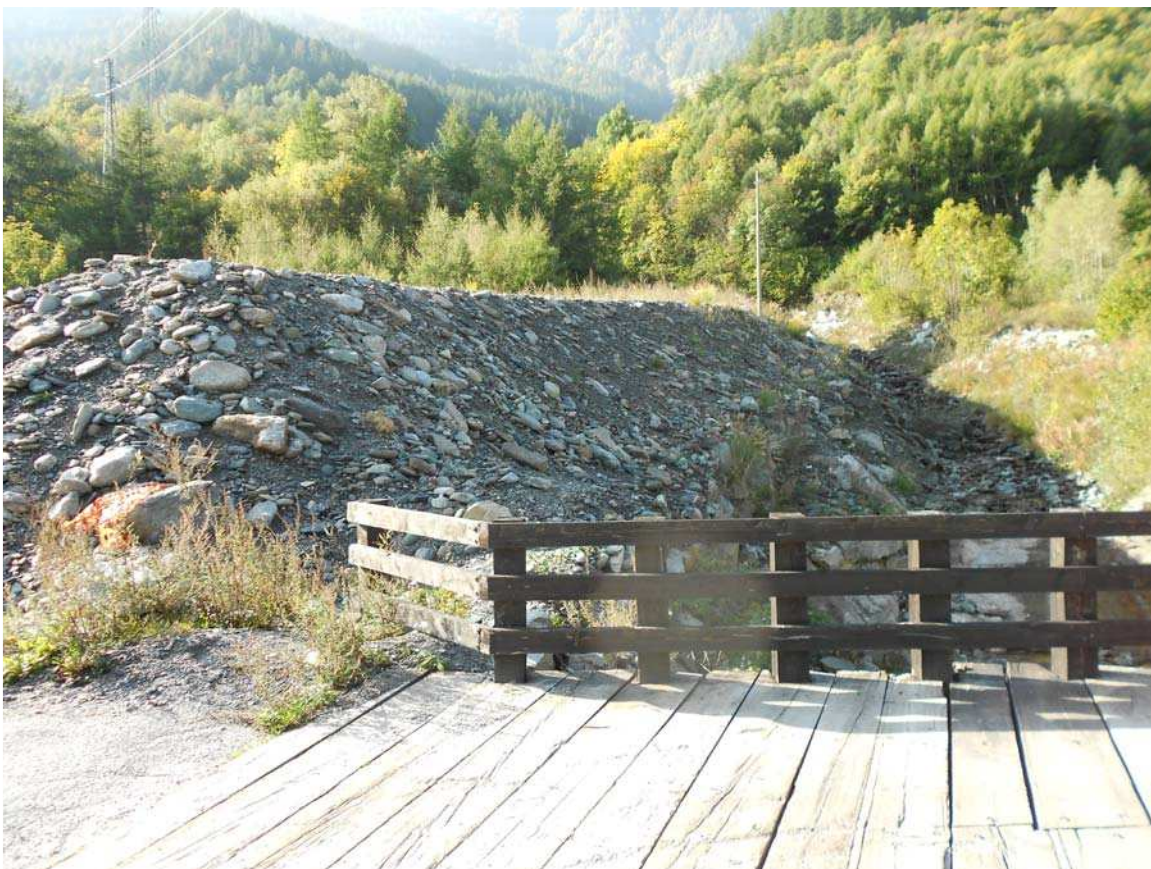
Foto 001 – Opera PAIRAR001 . Ripresa da valle.
